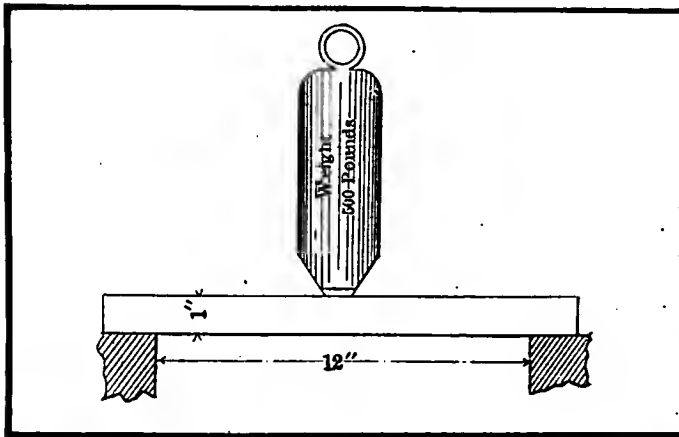
Fig. 1—Impact test
